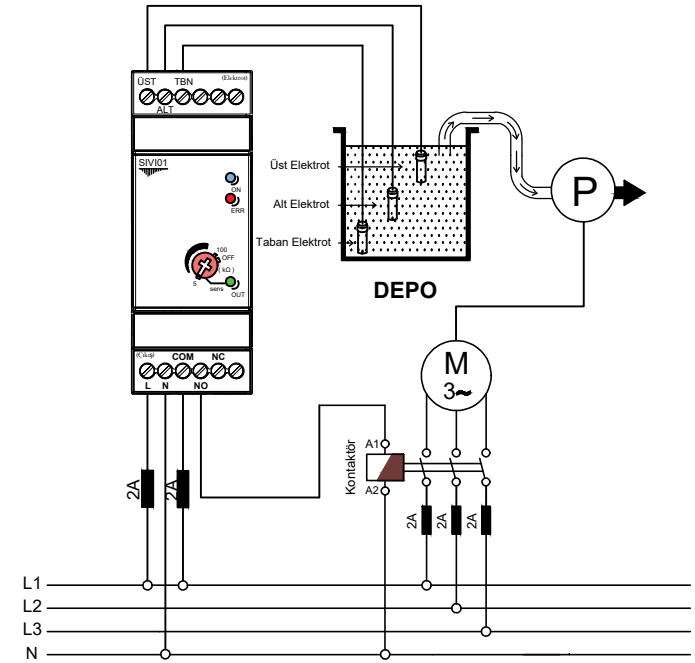
Depoyu Boşaltmak İçin Bağlantı Şeması
