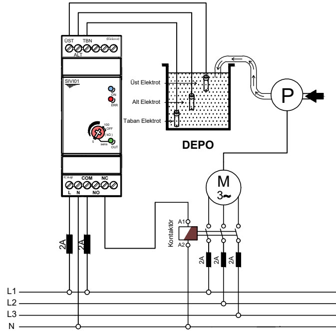
Depoyu Doldurmak İçin Bağlantı Şeması
